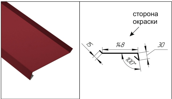
Отлив оконный
