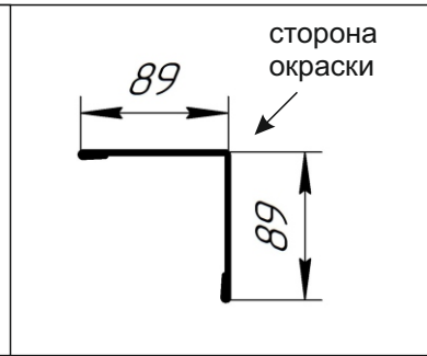
Угол внешний (Угол наружный)
