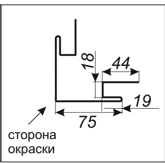
Угол внешний сложный
