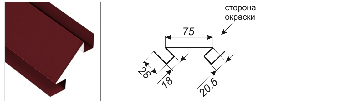
Угол внутренний сложный
