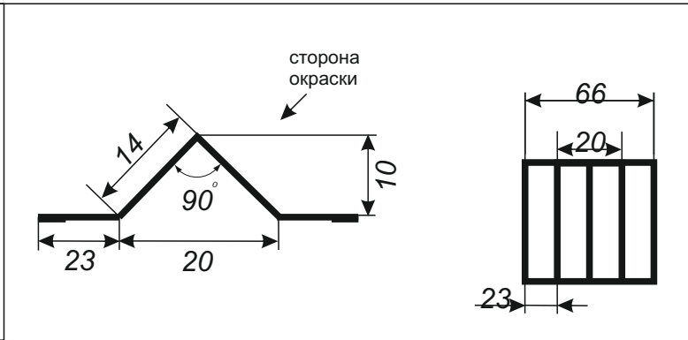
Крепежная планка «Усиленная»
