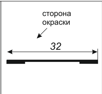
Завершающая планка «Домик»
