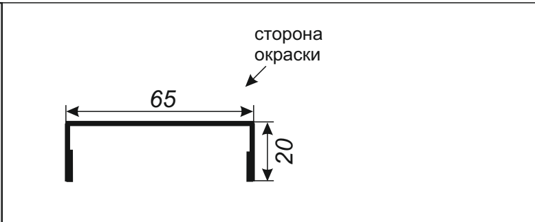
Крепежная планка «Усиленная»
