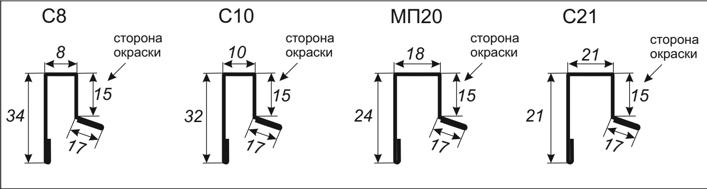
Верхняя планка для штакетника
