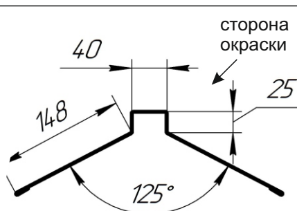
Фронтонная (торцевая) планка
