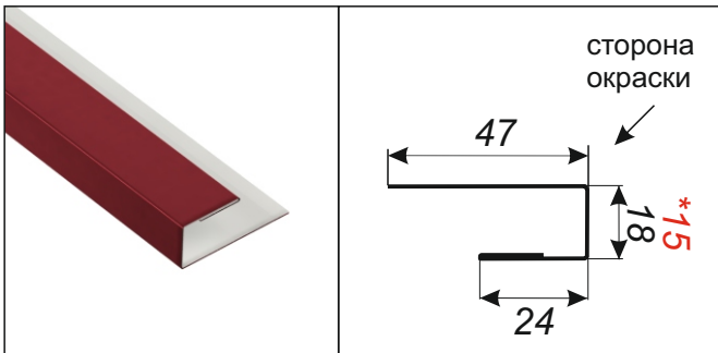
Отлив оконный
