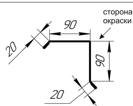
Фронтонная (торцевая) планка
