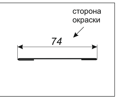
Планка стыковочная сложная (Н-профиль) и простая
