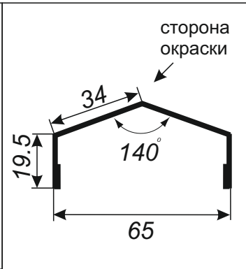
Завершающая планка «Домик»
