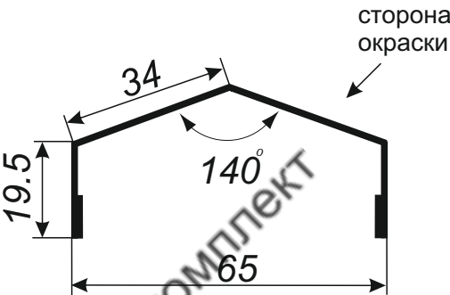
Завершающая планка «Домик»
