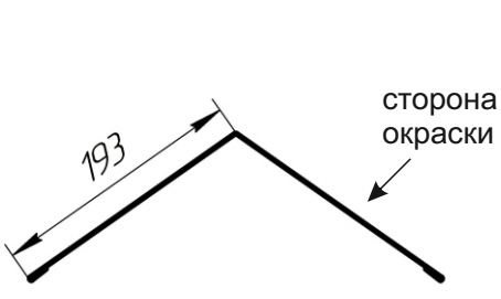
Конек фигурный Большой
