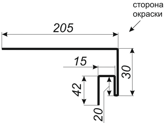
Планка околооконная (J-фаска)
