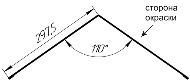
Накладка ендовы
