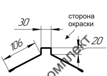
Ендова
