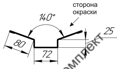
Фронтонная планка (Торцевая)
