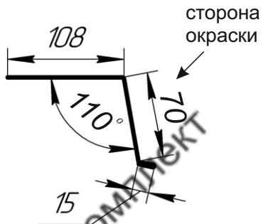
Карнизная планка
