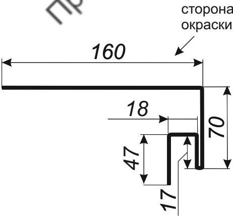
Планка окопосконная (J-фаска)
