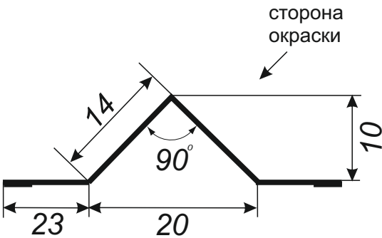
Крепежная планка «Усиленная»
