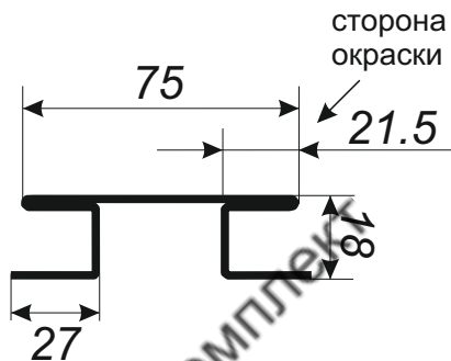
Планка стыковочная сложная (H-профиль)
