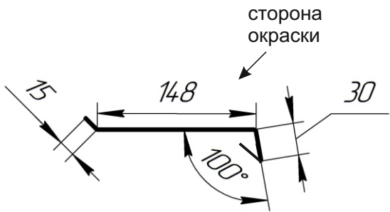
Угол внутренний сложный
