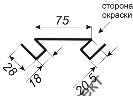
J-профиль
