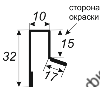
Верхняя планка С10
