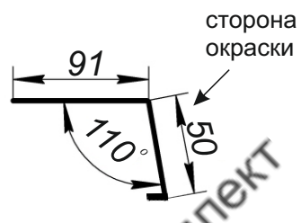
Капельник
