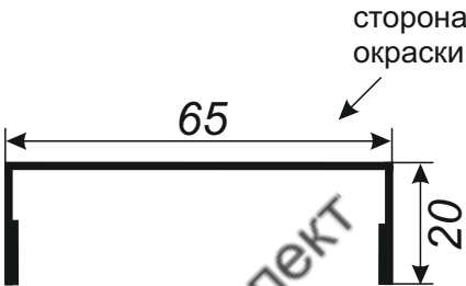
Завершающая планка
