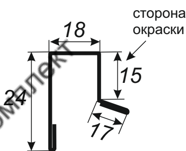
Верхняя планка МП20/С20
