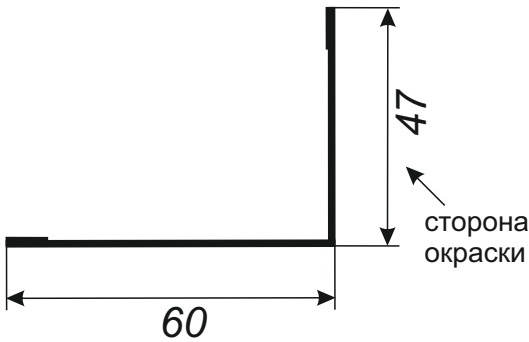
Завершающая планка
