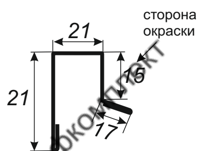
Верхняя планка С21
