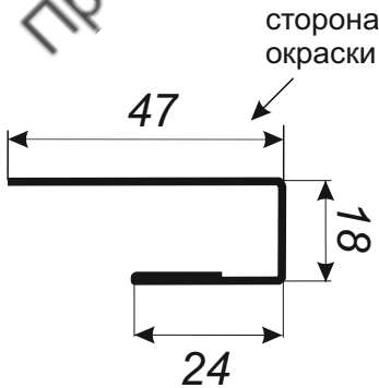
J-профиль
