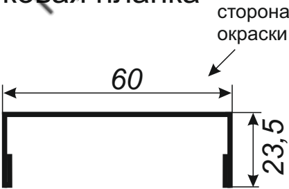
Боковая планка
