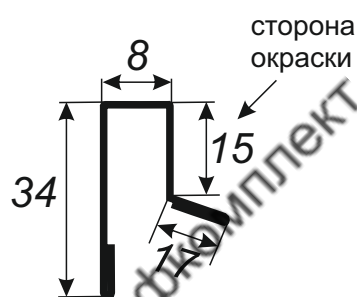
Верхняя планка С8
