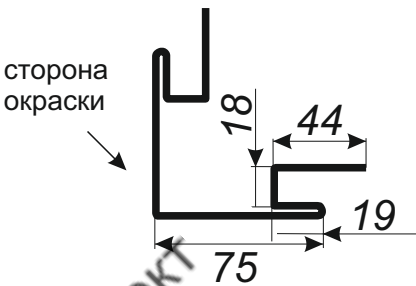
Планка стыковочная
