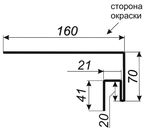
Планка околооконная (J-фаска)
