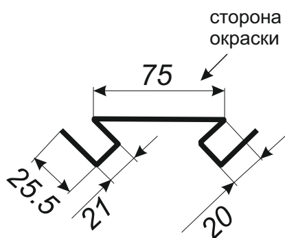
Угол внутренний сложный
