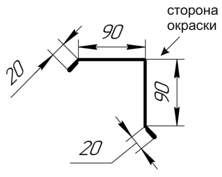
Фронтонная планка (Торцевая)
