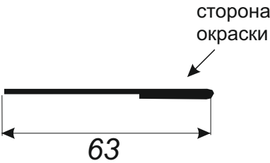
Планка завершающая
