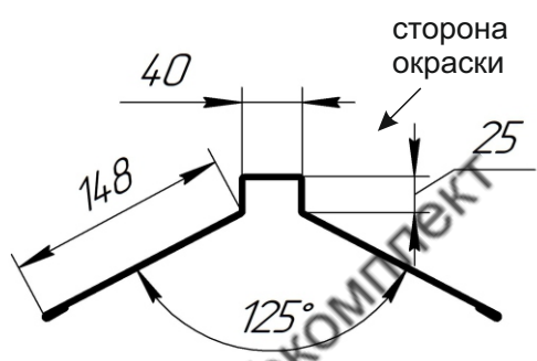
Конек фигурный Большой
